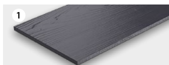
HardiePlank® Holzstruktur Maße: 3.600 x 180 x 8 mm
